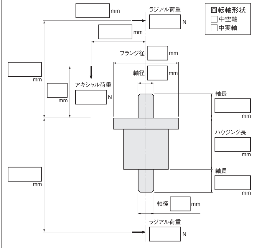
荷重・概略寸法図
